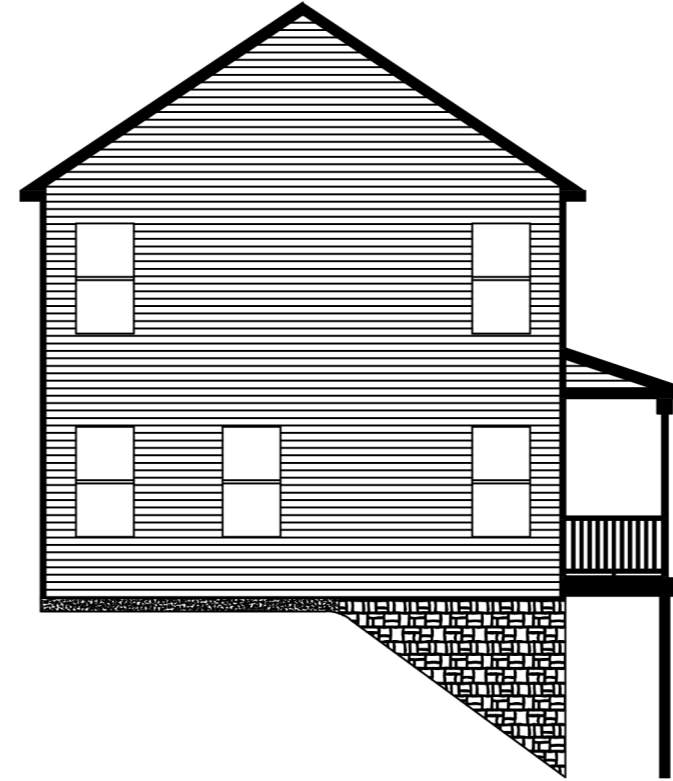
Elevation - Right
